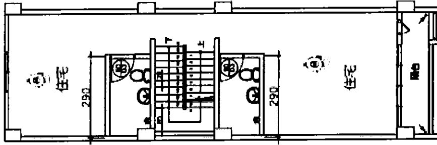
貳層平面圖
