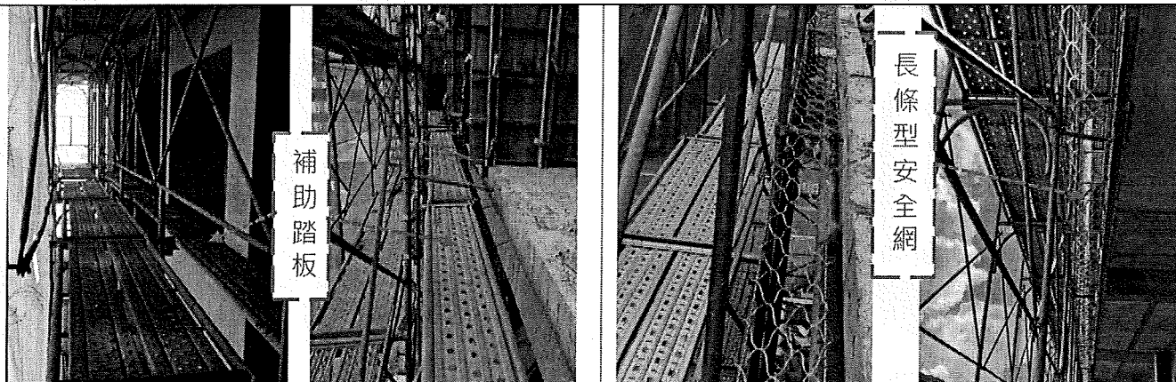
施工架工作臺與建築物間隙大於 20 公分時，應設置補助踏板或長條型安全網。
