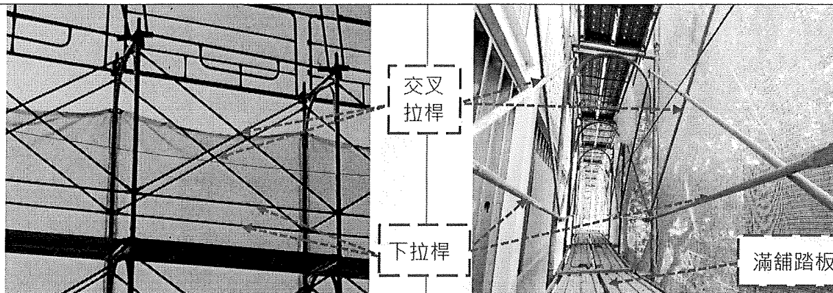
施工架工作臺應設置內外兩側交叉拉桿、下拉桿；工作臺寬度應大於 40 公分且鋪滿密接之踏板。
