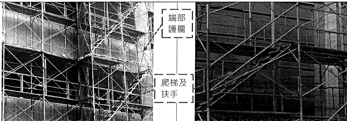
施工架工作臺端部開口部分應設置護欄及設置安全上下設備(爬梯)，並於爬梯設置護欄(扶手)。
