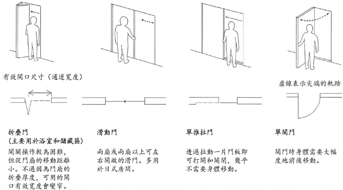
圖 5-1 門類型
