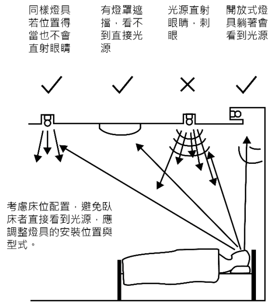
圖 3-44 頭頂照明
