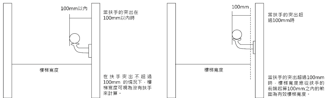
圖 3-17 樓梯寬度
