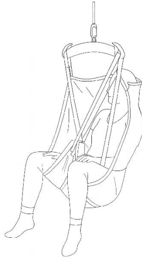
圖 5-33 分腿高背、網狀吊帶使用情境圖 (資料來源：本研究繪製)
