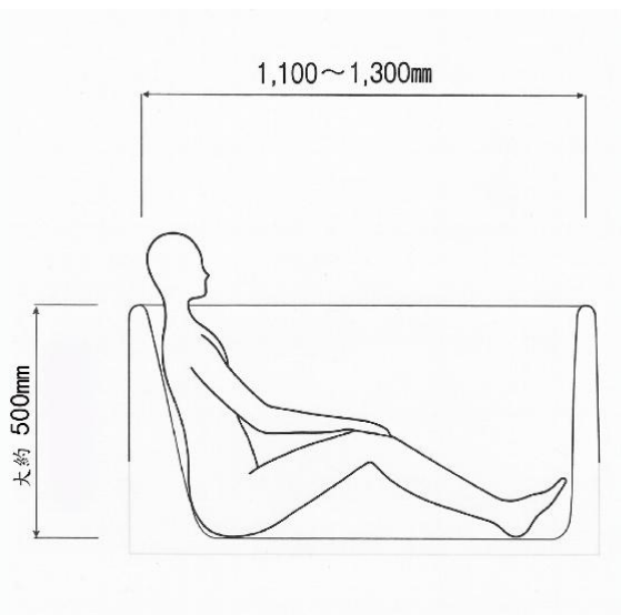
圖 5-5 西式浴缸
