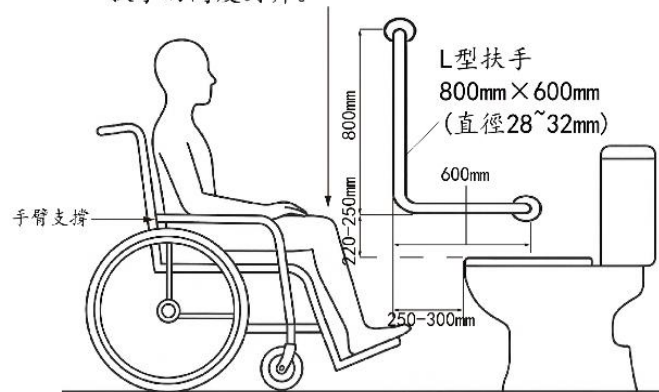
圖 5-4 馬桶扶手安裝高度 (資料來源：本研究繪製)
