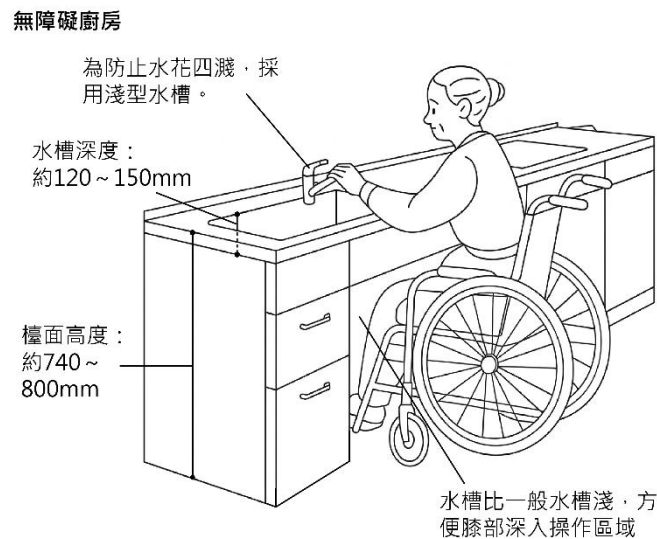
圖 3-41 可讓輪椅進出的廚房
