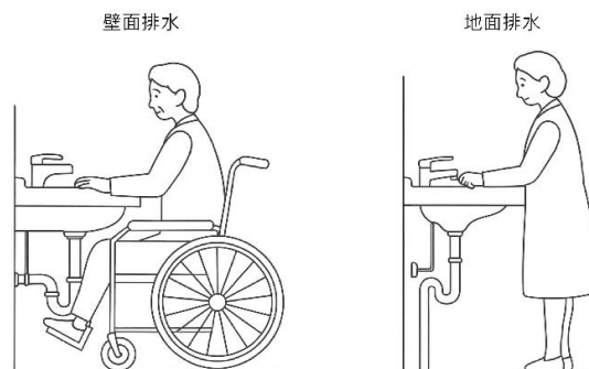
圖 3-37 洗臉盆檯面下方的水管
