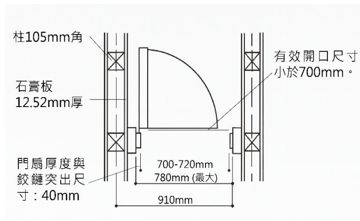
圖 3-8 有效開口尺寸 (資料來源：本研究繪製)
